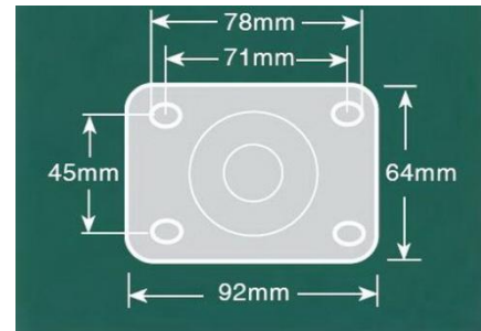
Kích thước tâm lắp
